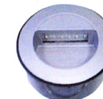
W91492 1W 220V IP44 h=162 w=98
