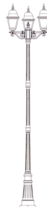
79910B S M L h=2730 2778 2740 h=3010 3058 3020
