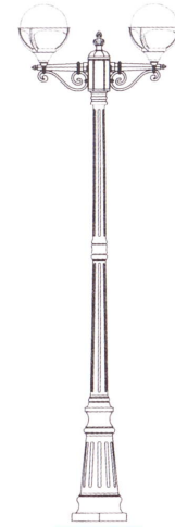
88109A h=2230
